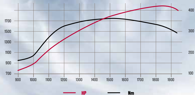
TOČIVÝ MOMENT V MN, S396 A S416
